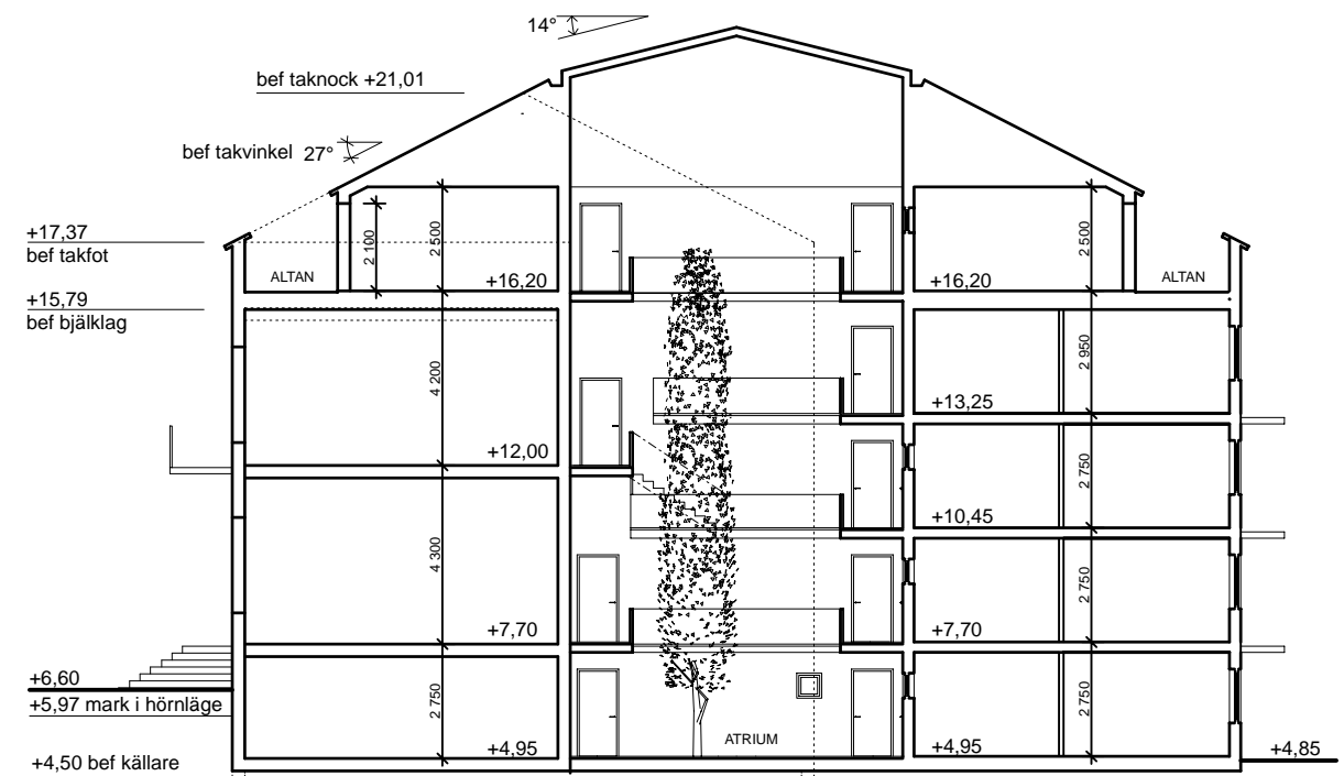
PRINCIPSEKTION SKALA 1:200
