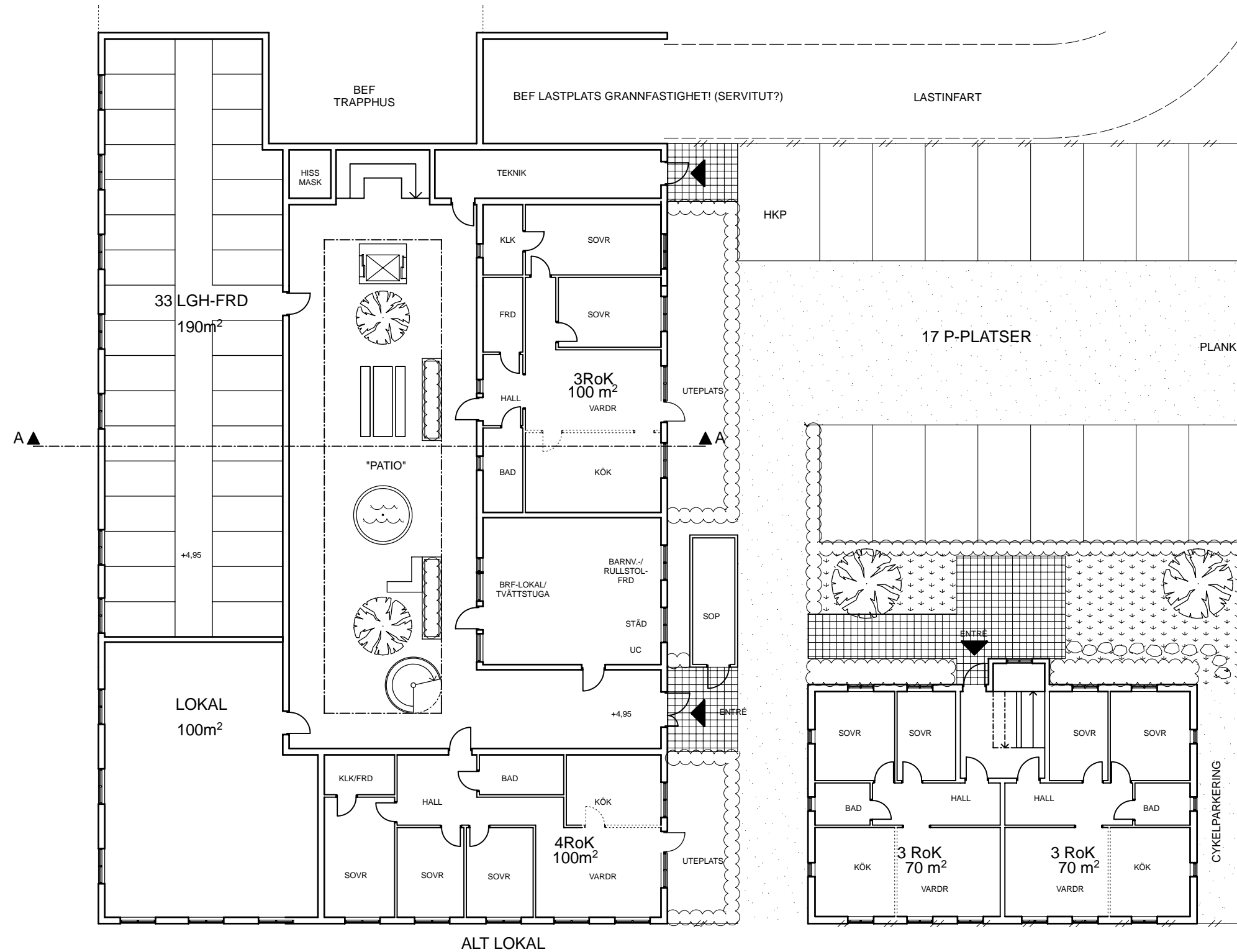
NEDRE ENTRÉPLAN +4,95 SKALA 1:200
