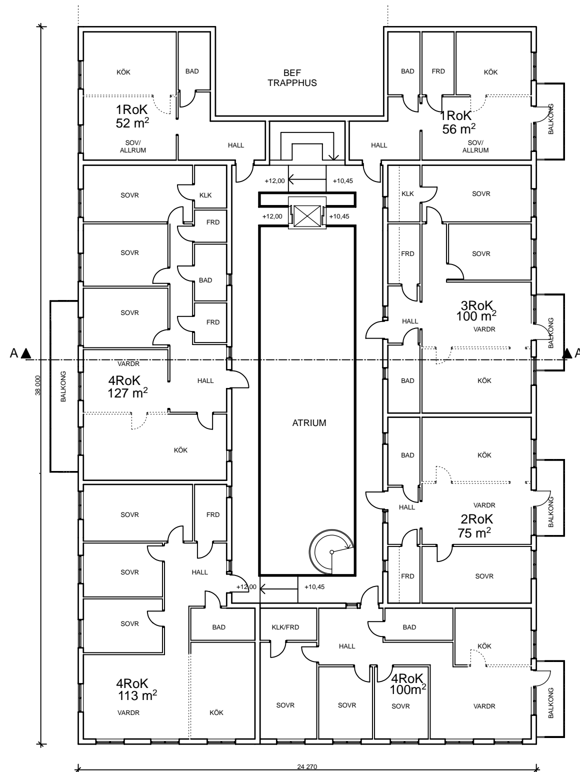
TYPPLAN SKALA 1:200
